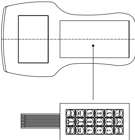
Draufsicht Oberschale Top part Top view
