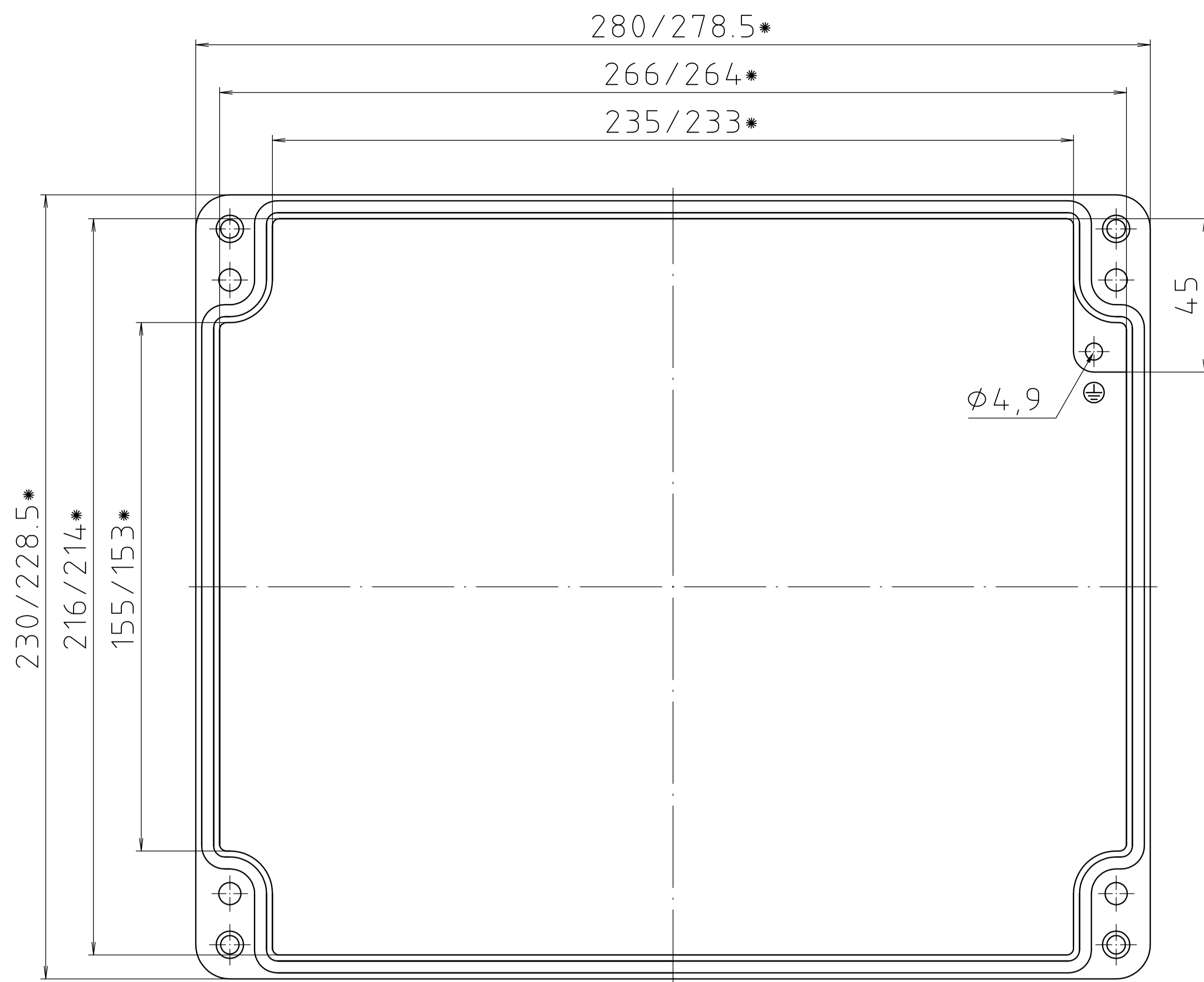
Deckel / lid
