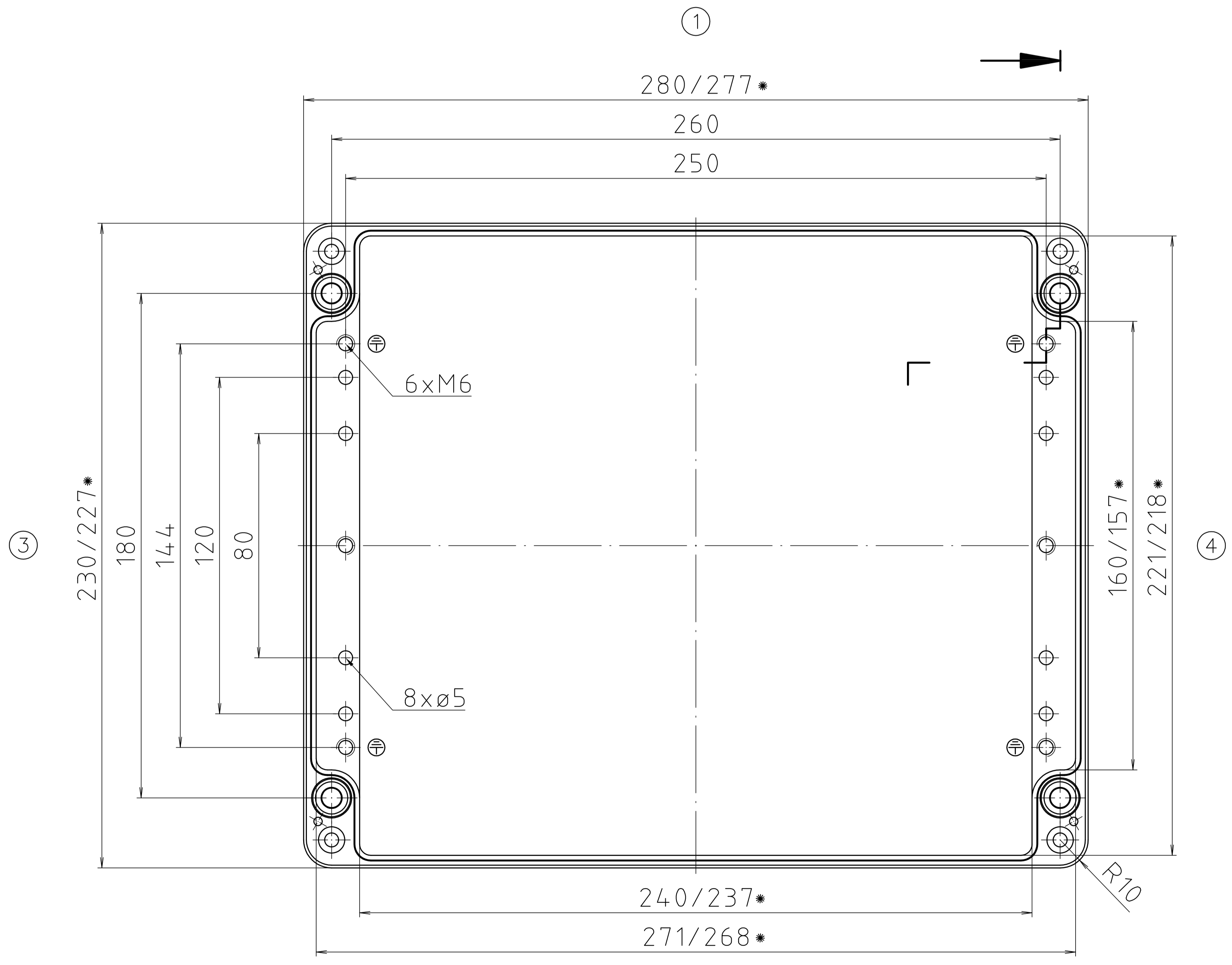
Unterteil / base
