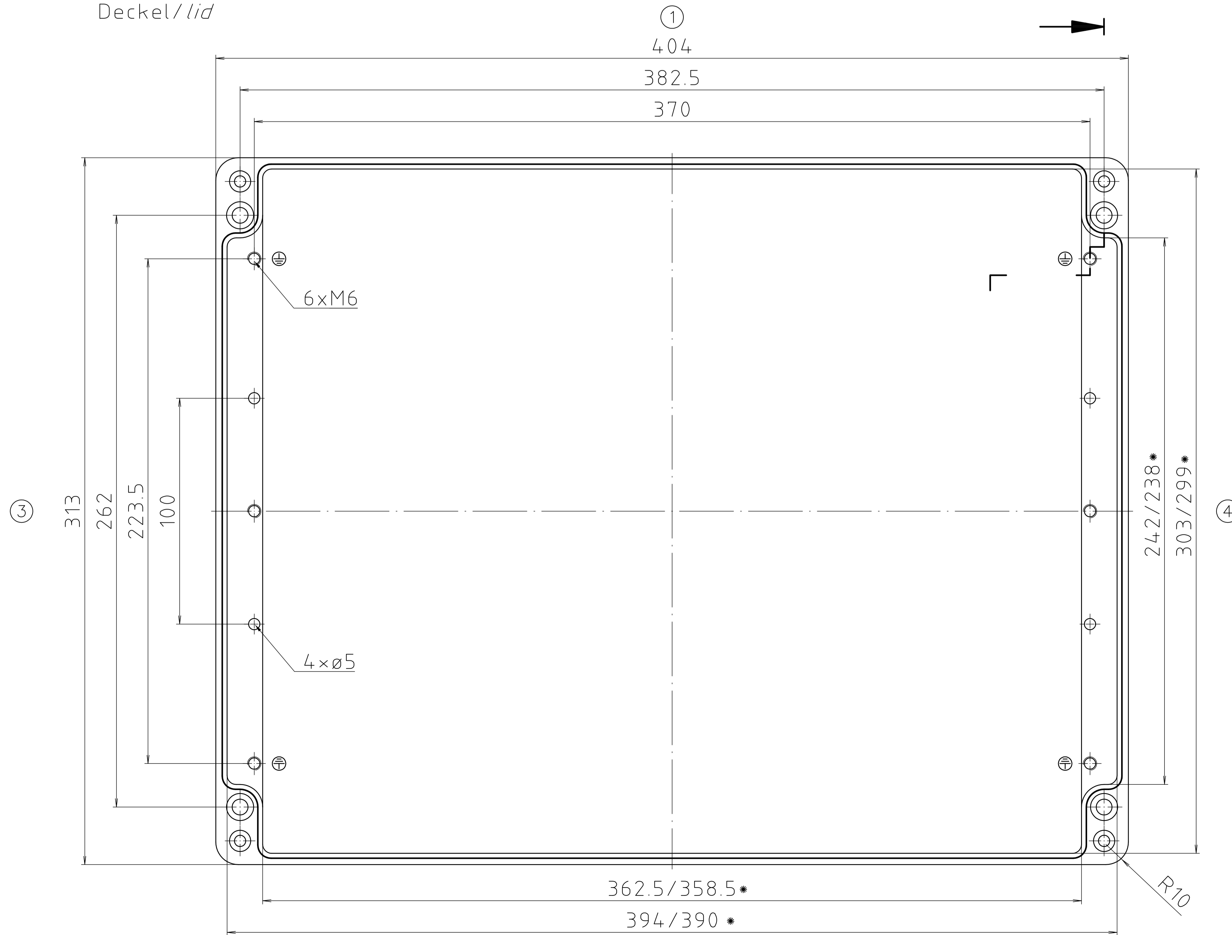
Unterteil / base
