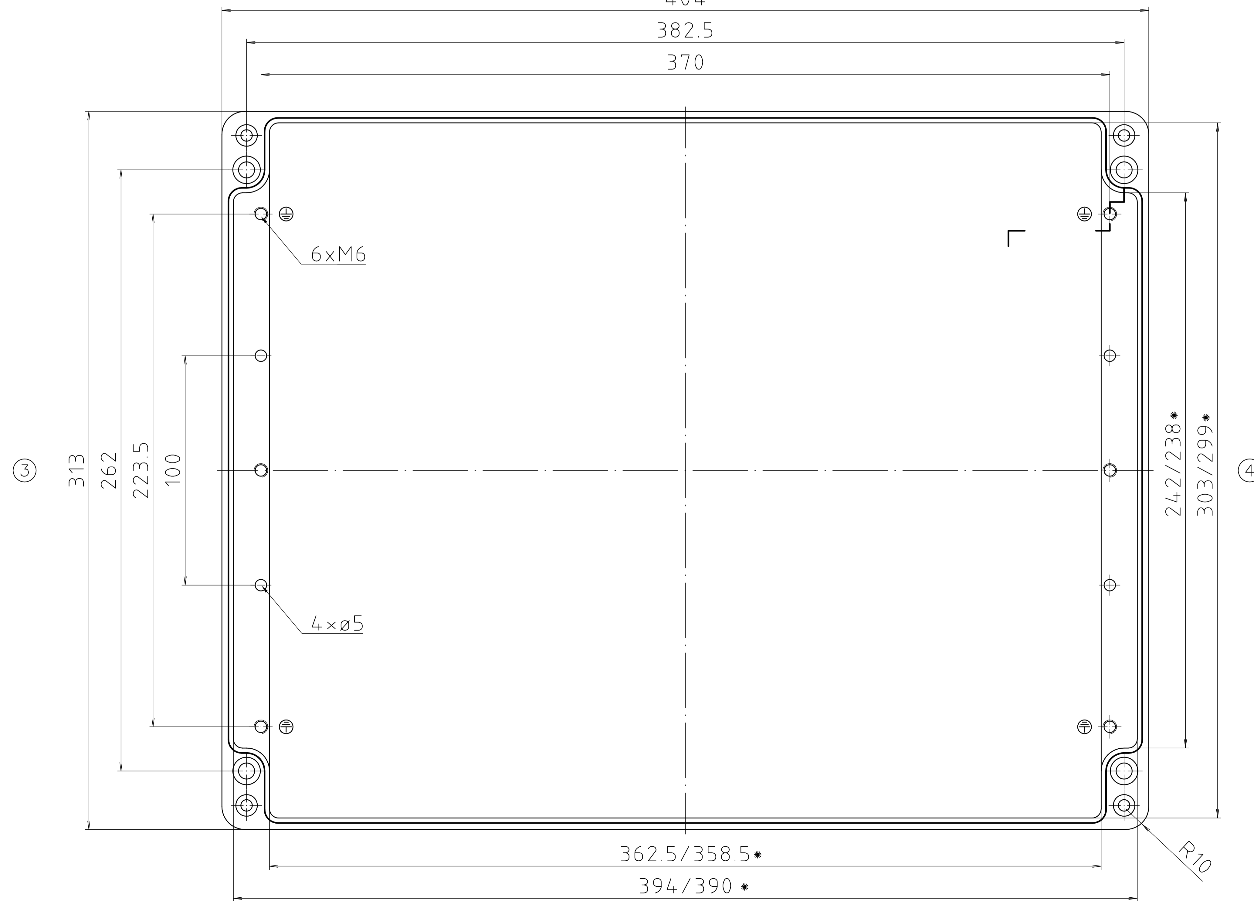
Unterteil / base
