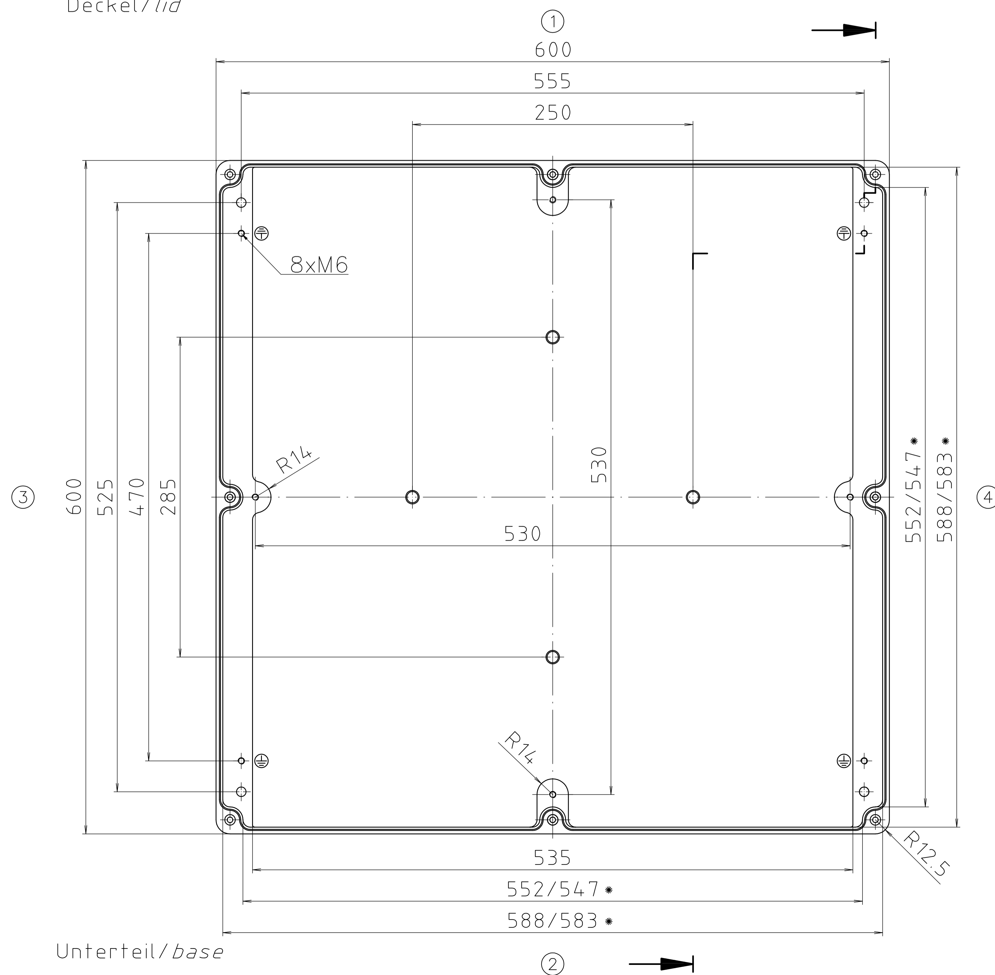
Deckel / lid
