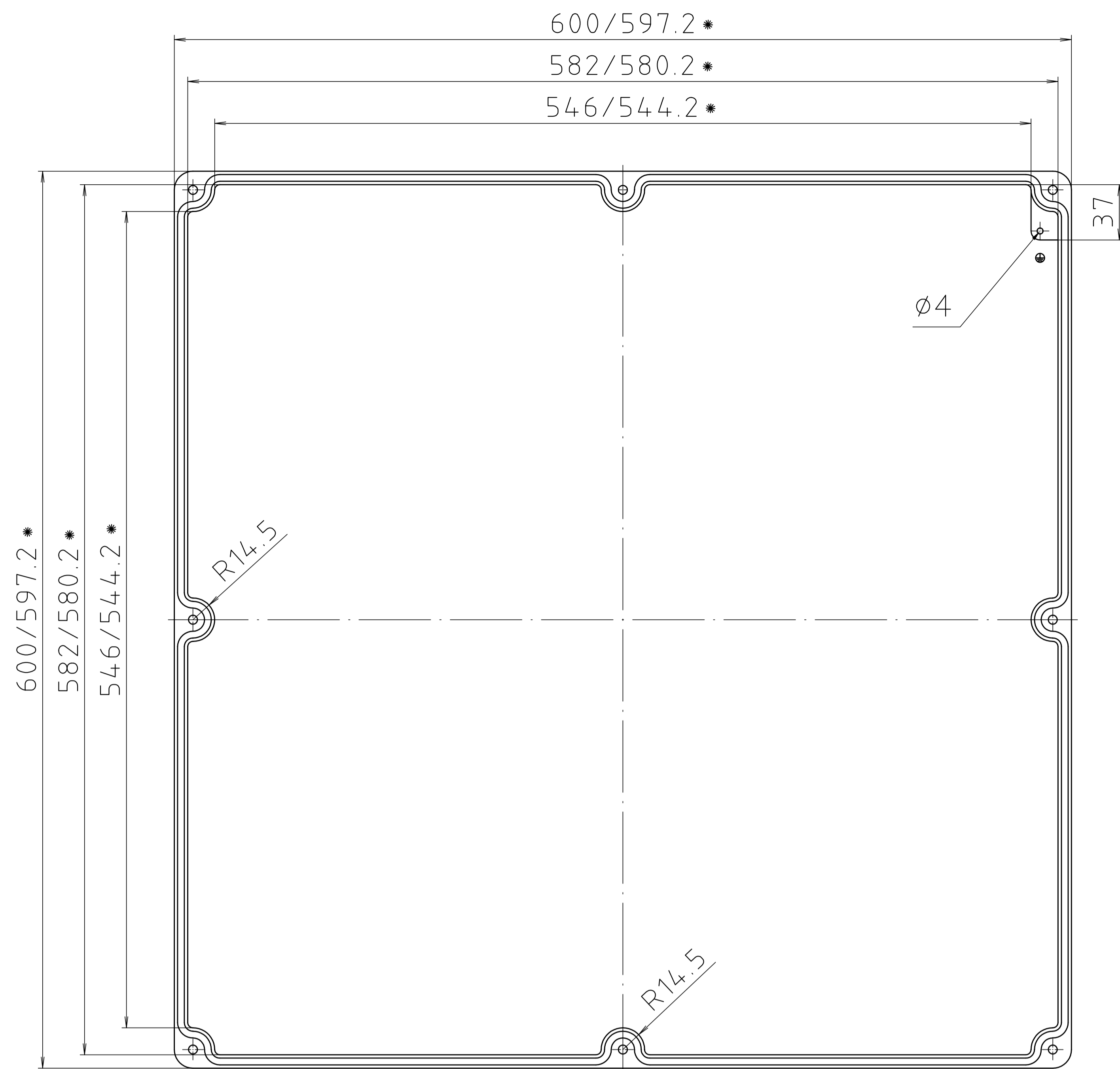
Deckel / lid
