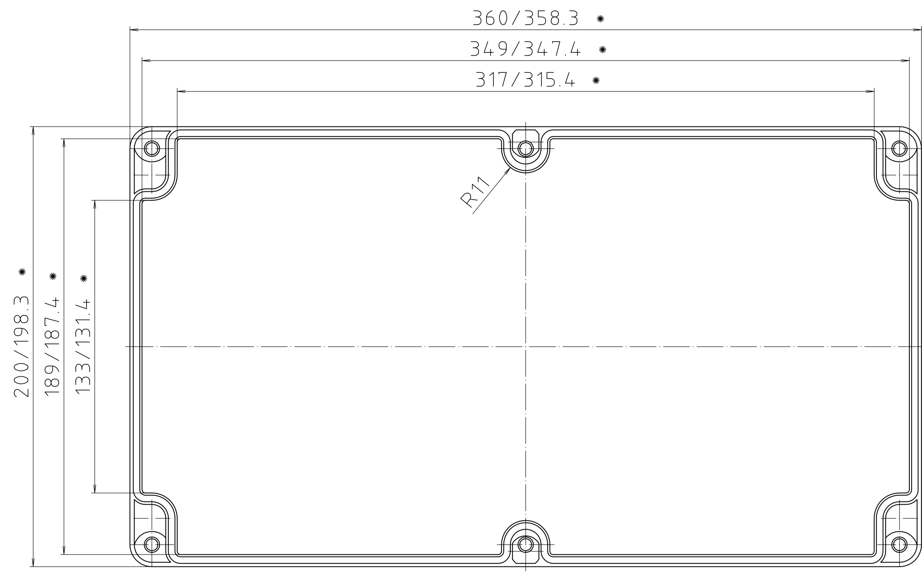
Deckel / lid
