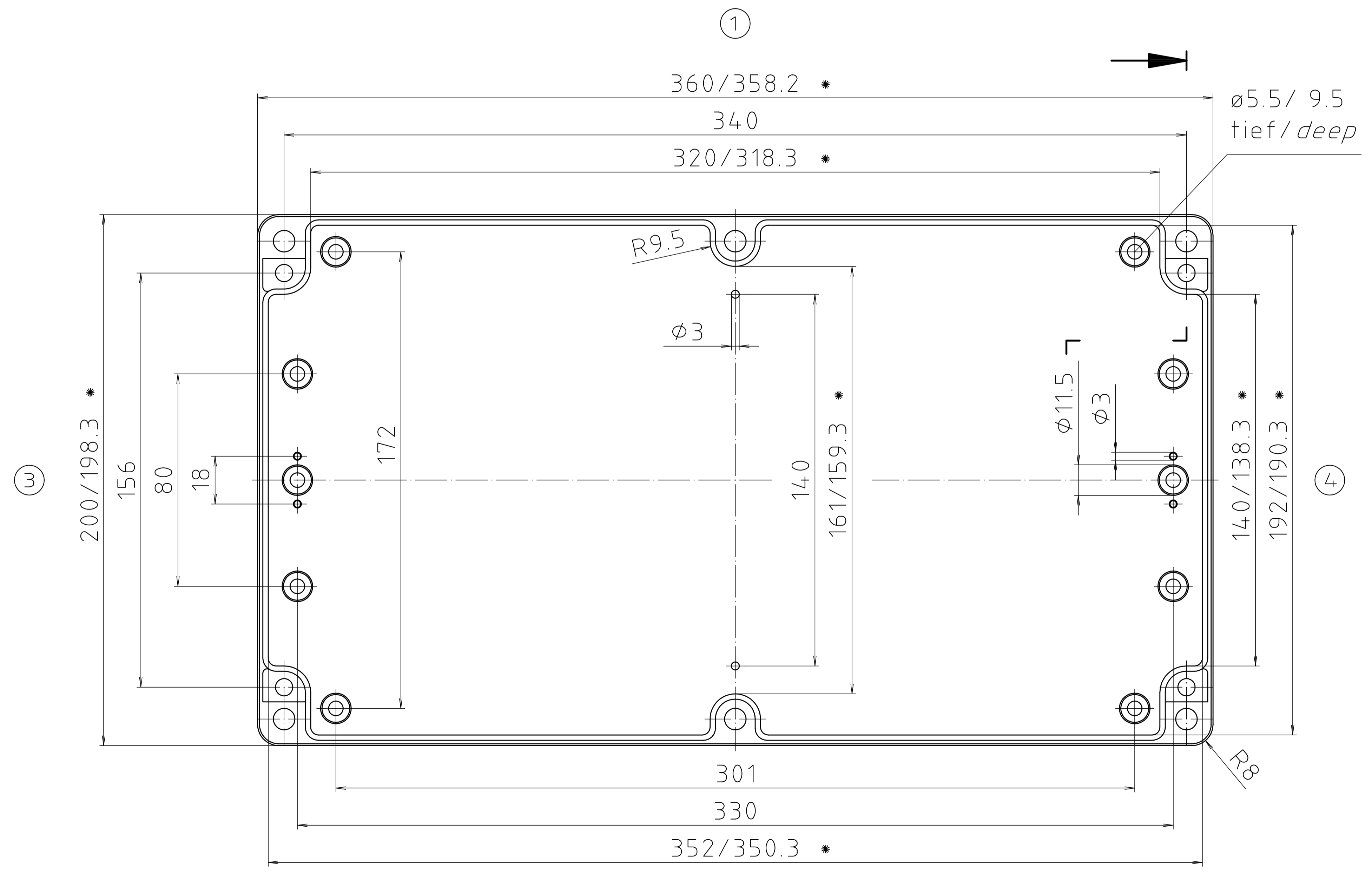
Unterteil / base
