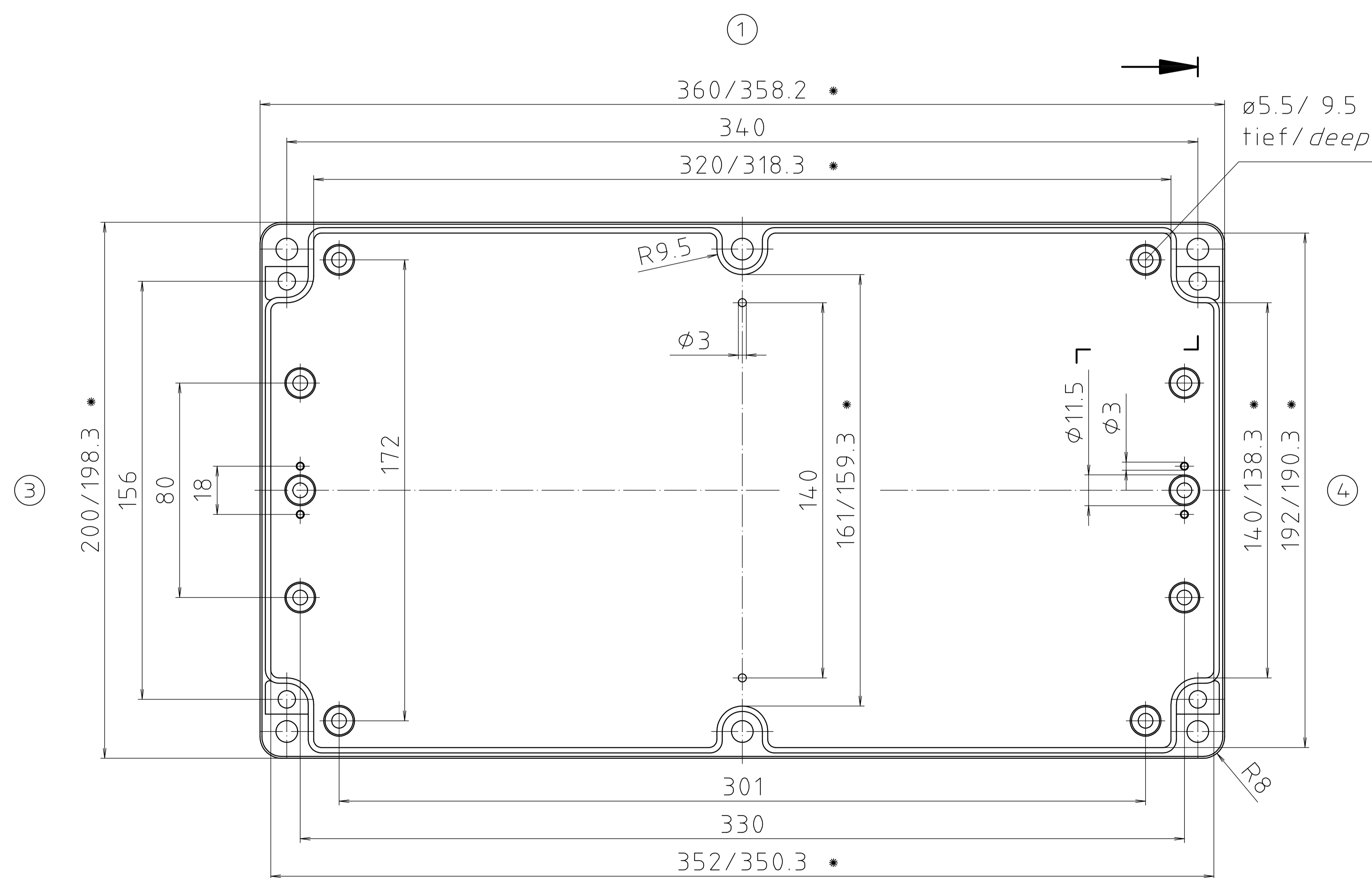
Unterteil/base
