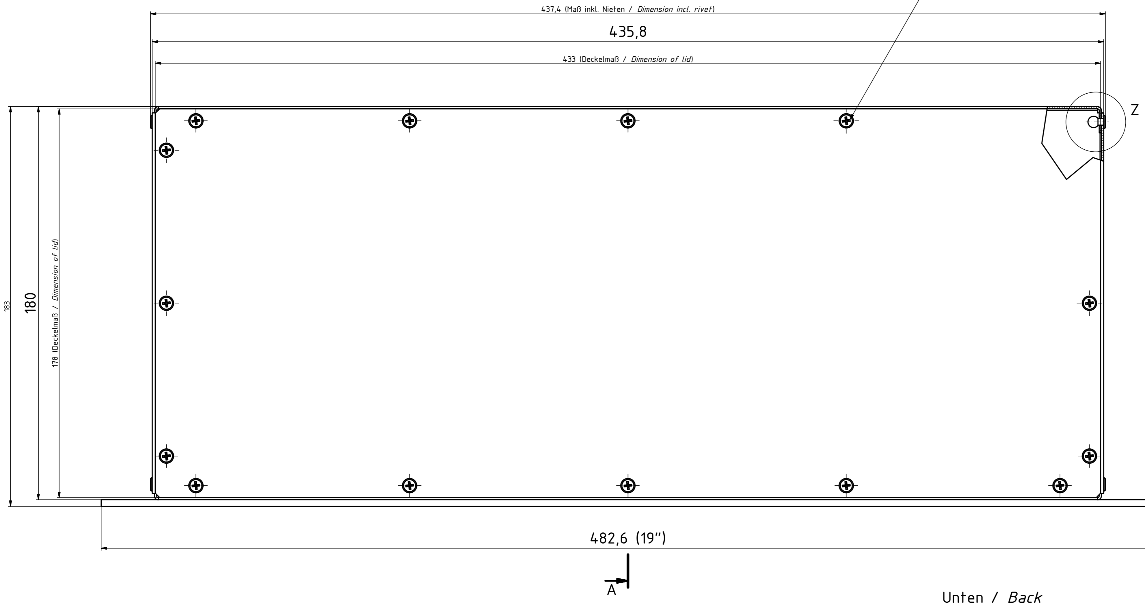
Rückansicht / Rear view
