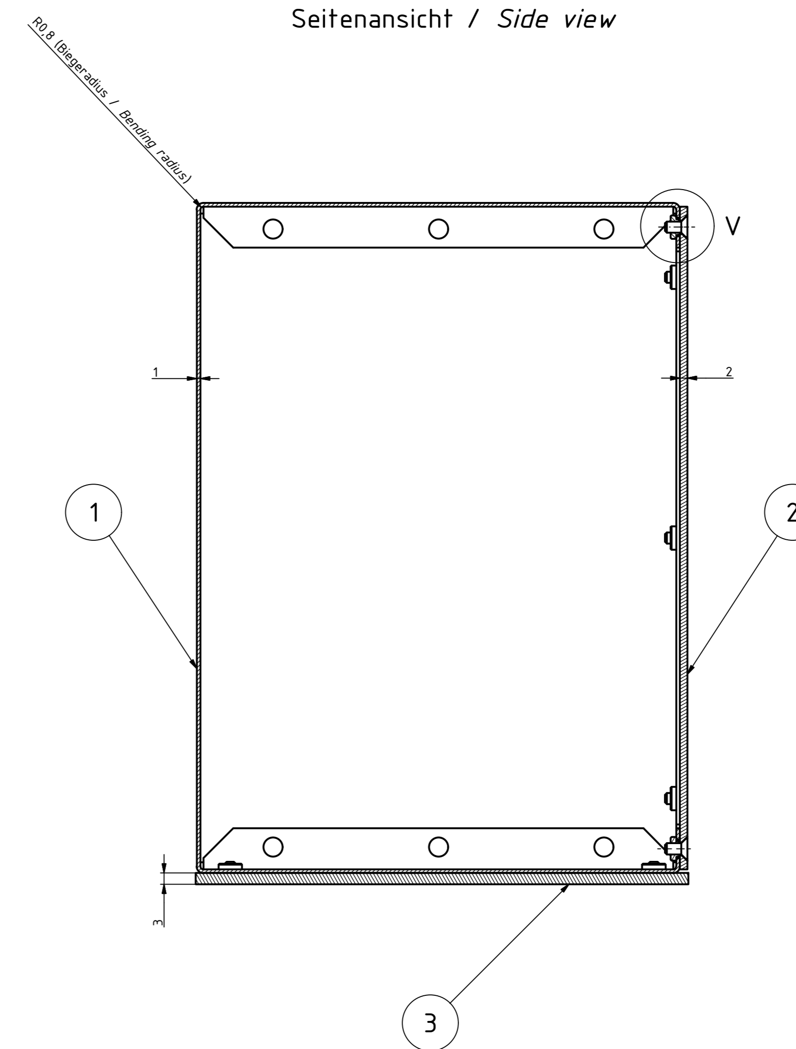
A-A ( 1 : 1 ) Seitenansicht / Side view
