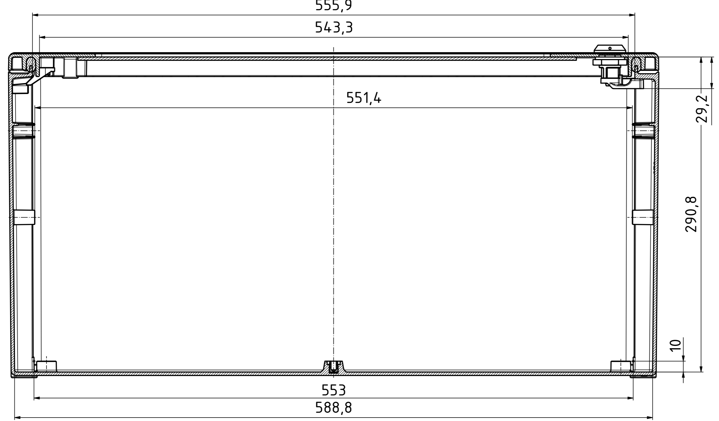
A-A ( 1 : 2 )
