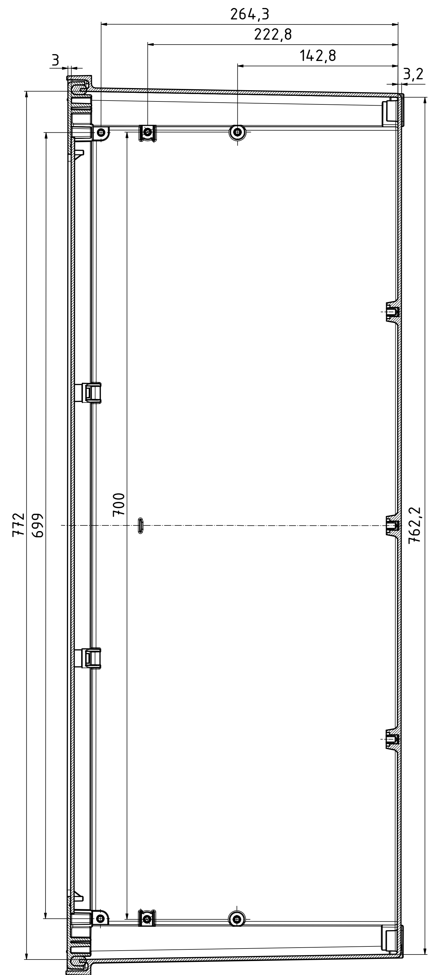
ISO ( 1 : 5 )
