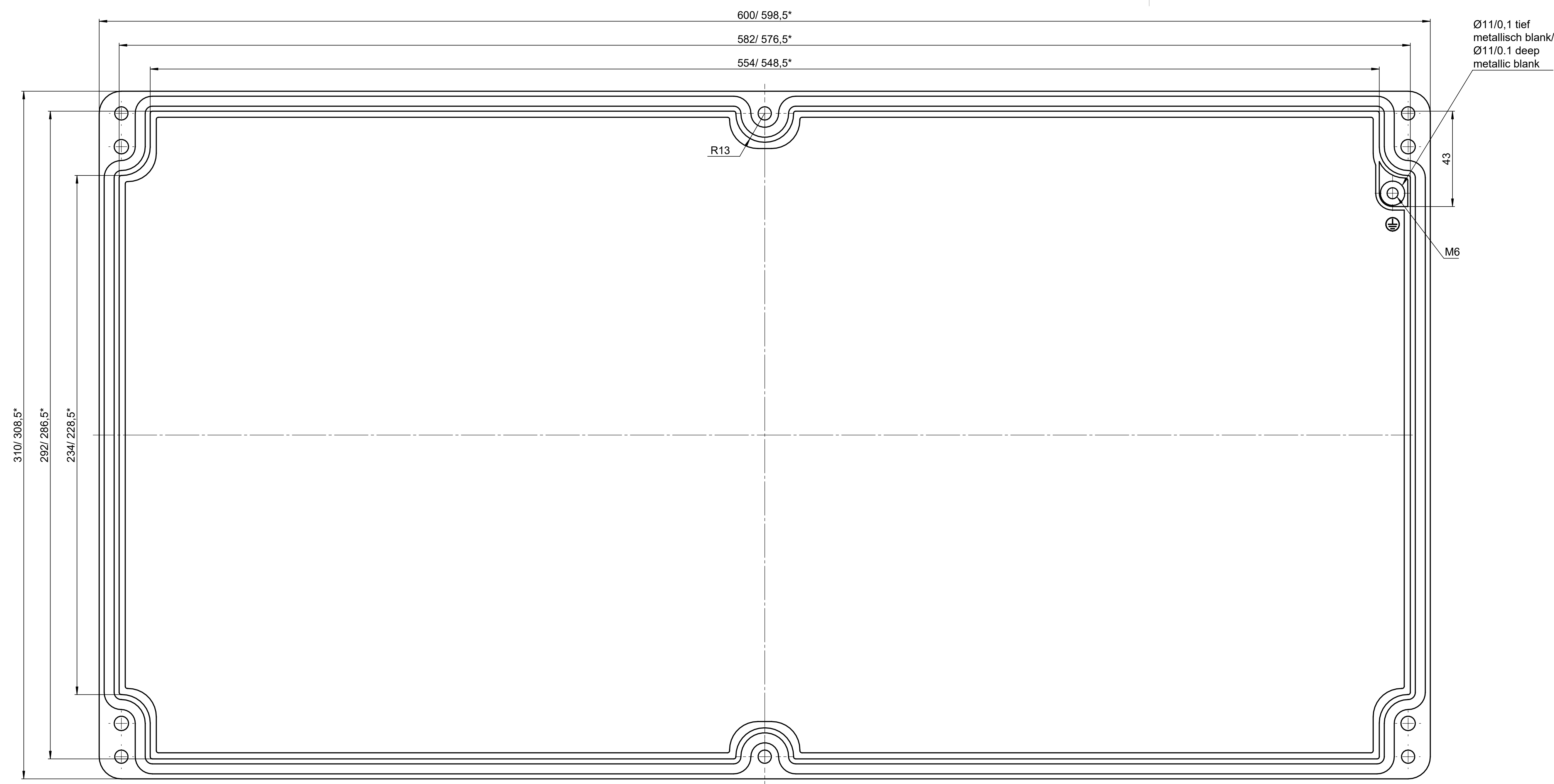
Deckel / Lid
