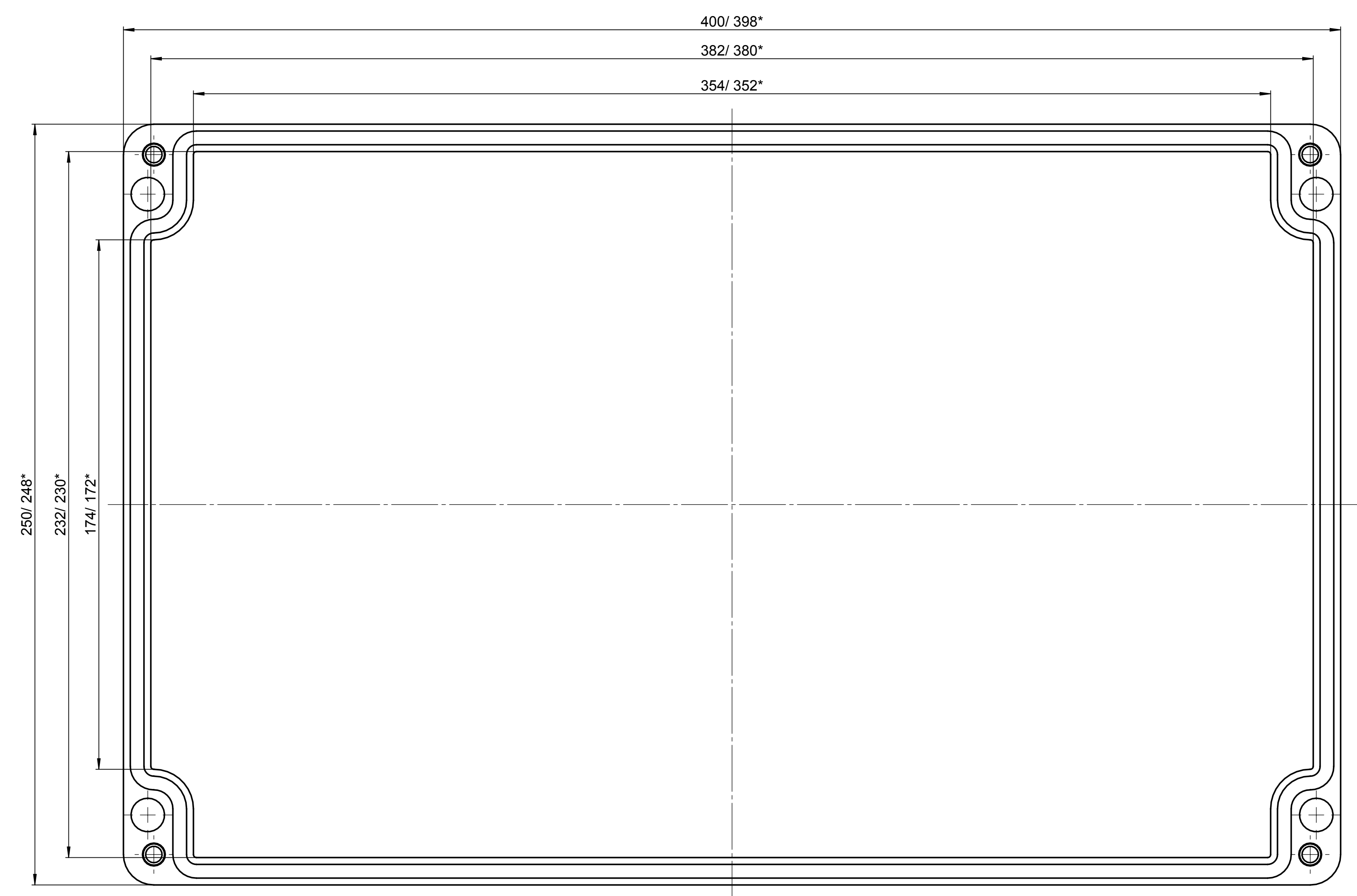
Deckel / Lid
