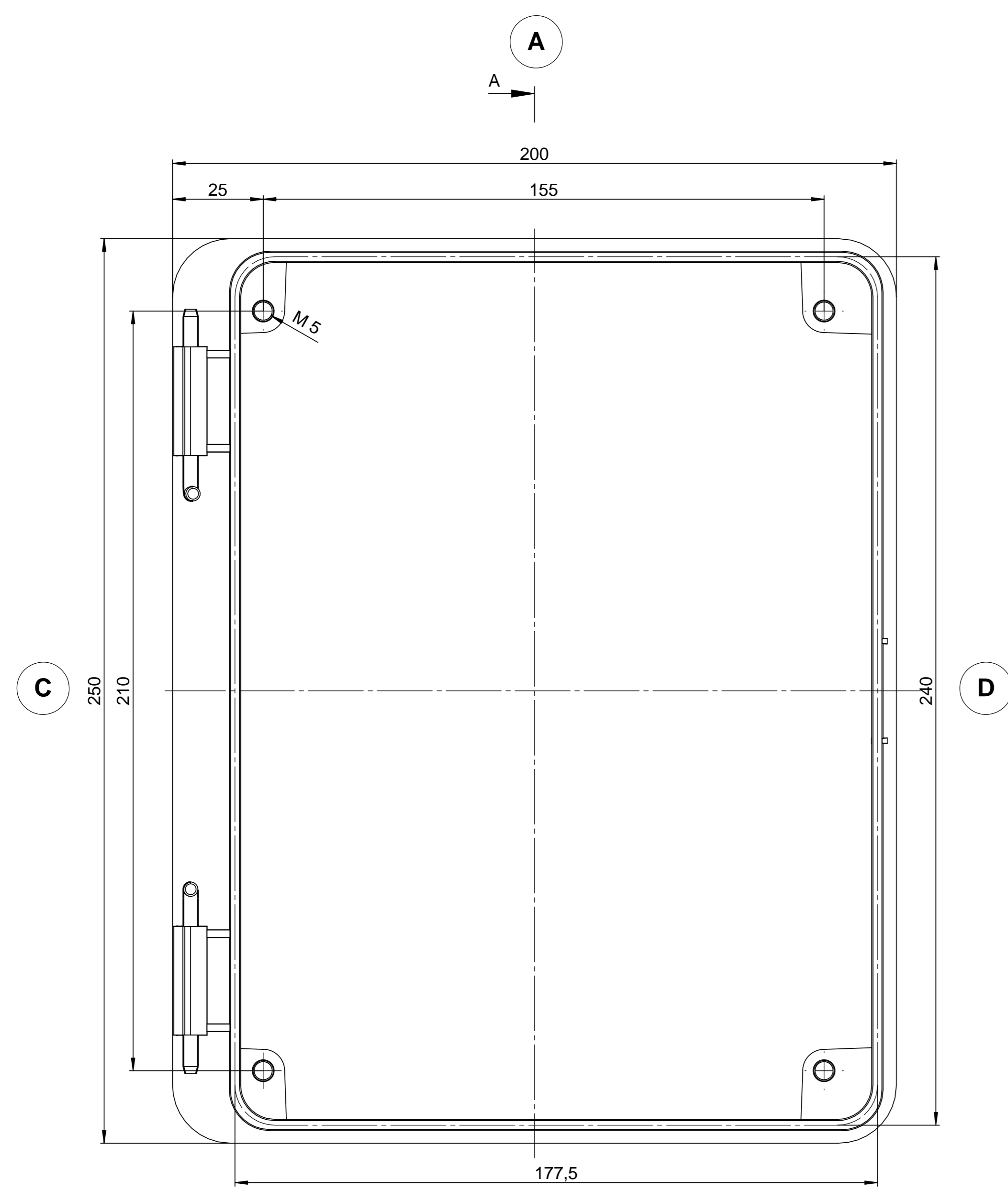
Unterteil
