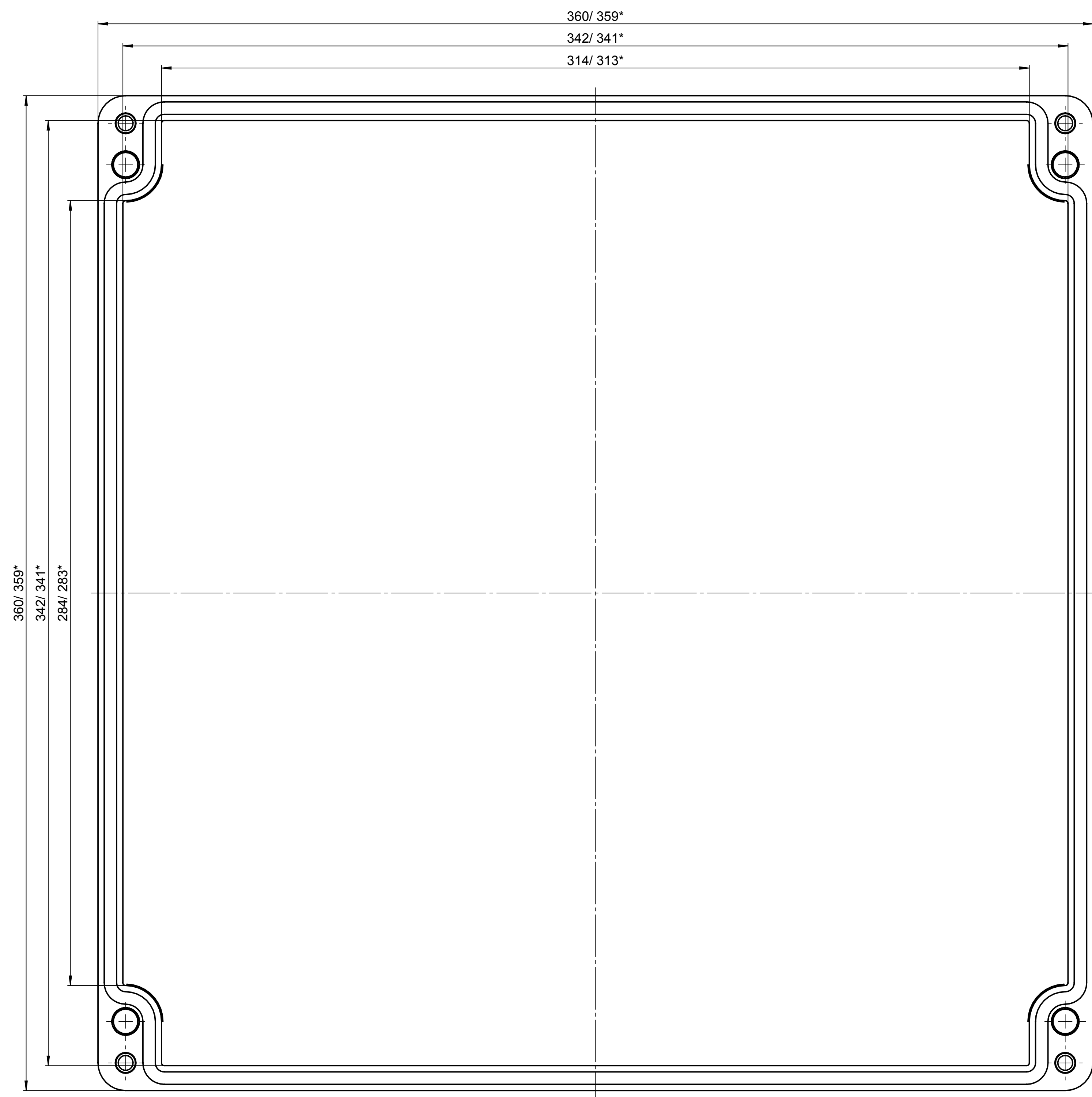
Deckel / Lid
