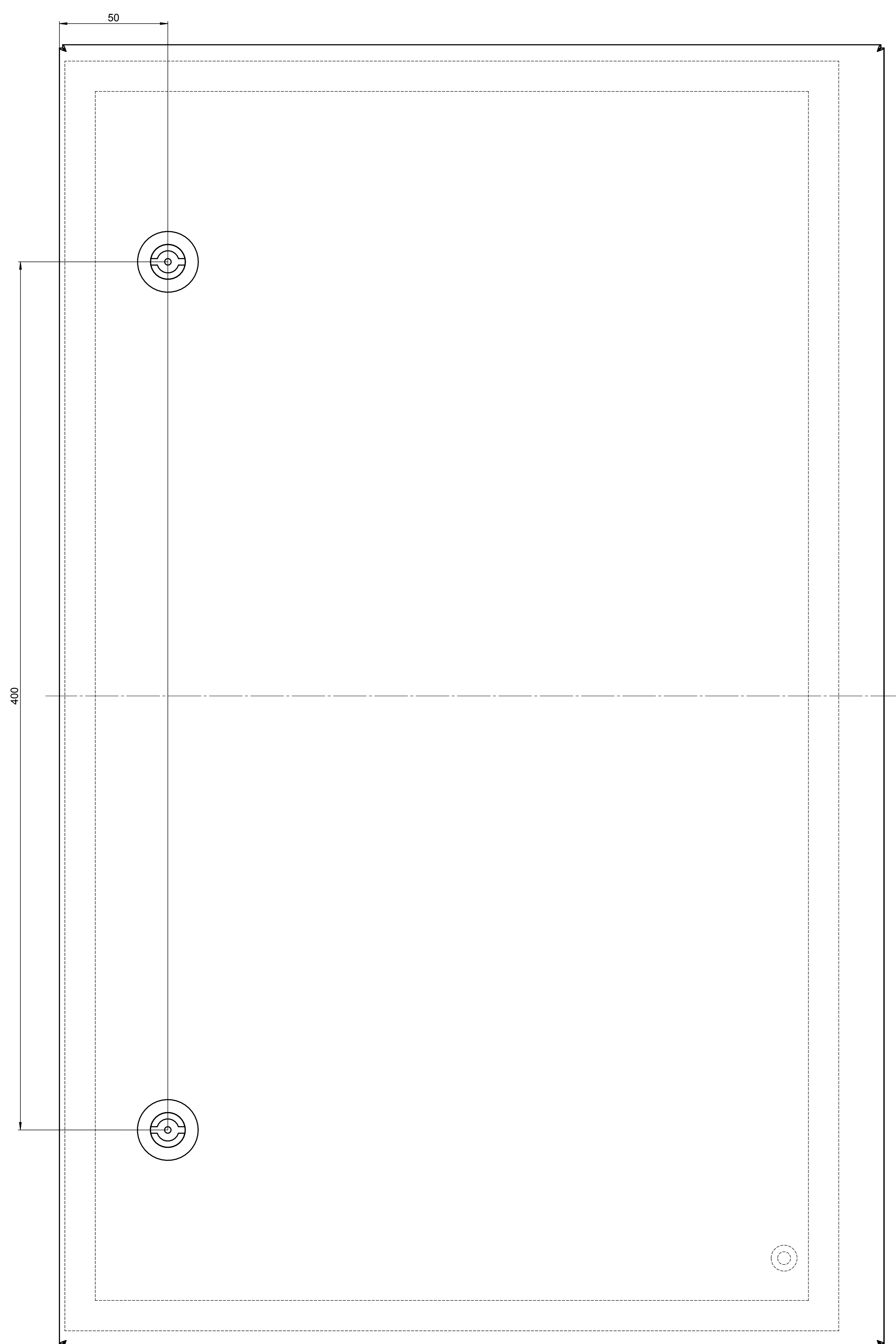
Deckeldraufsicht/ lid top view
