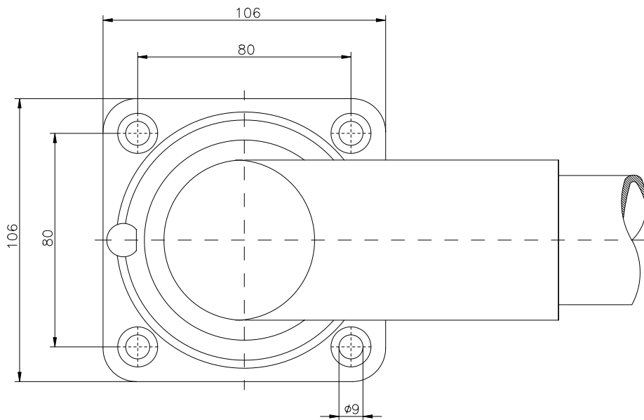
Aufsatzgelenk GT 48/2 Bestell-Nr. 49.49 66 00
