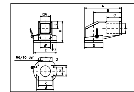
Flanschwinkelkupplung GT 50/2_60/2_80/2 Bestell-Nr. 49.517800 Bestell-Nr. 49.617800 Bestell-Nr. 49.817800
