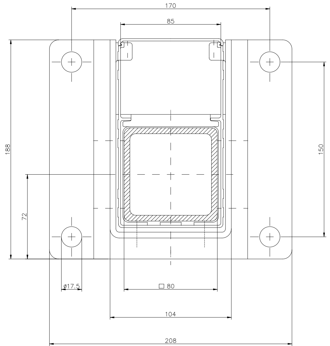
Standfuss/ Wandflansch Bestell-Nr.: 49.907401
