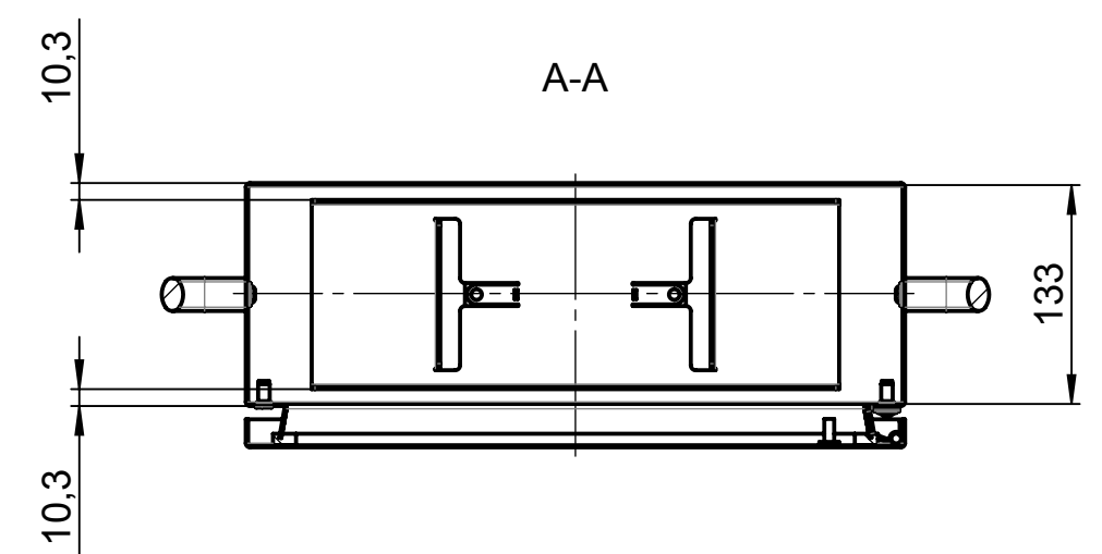
Verstärkerplatte an Seite A oder B, je nach Kupplungsbohrung reinforcing plate on side A or B, depending on coupling bore
