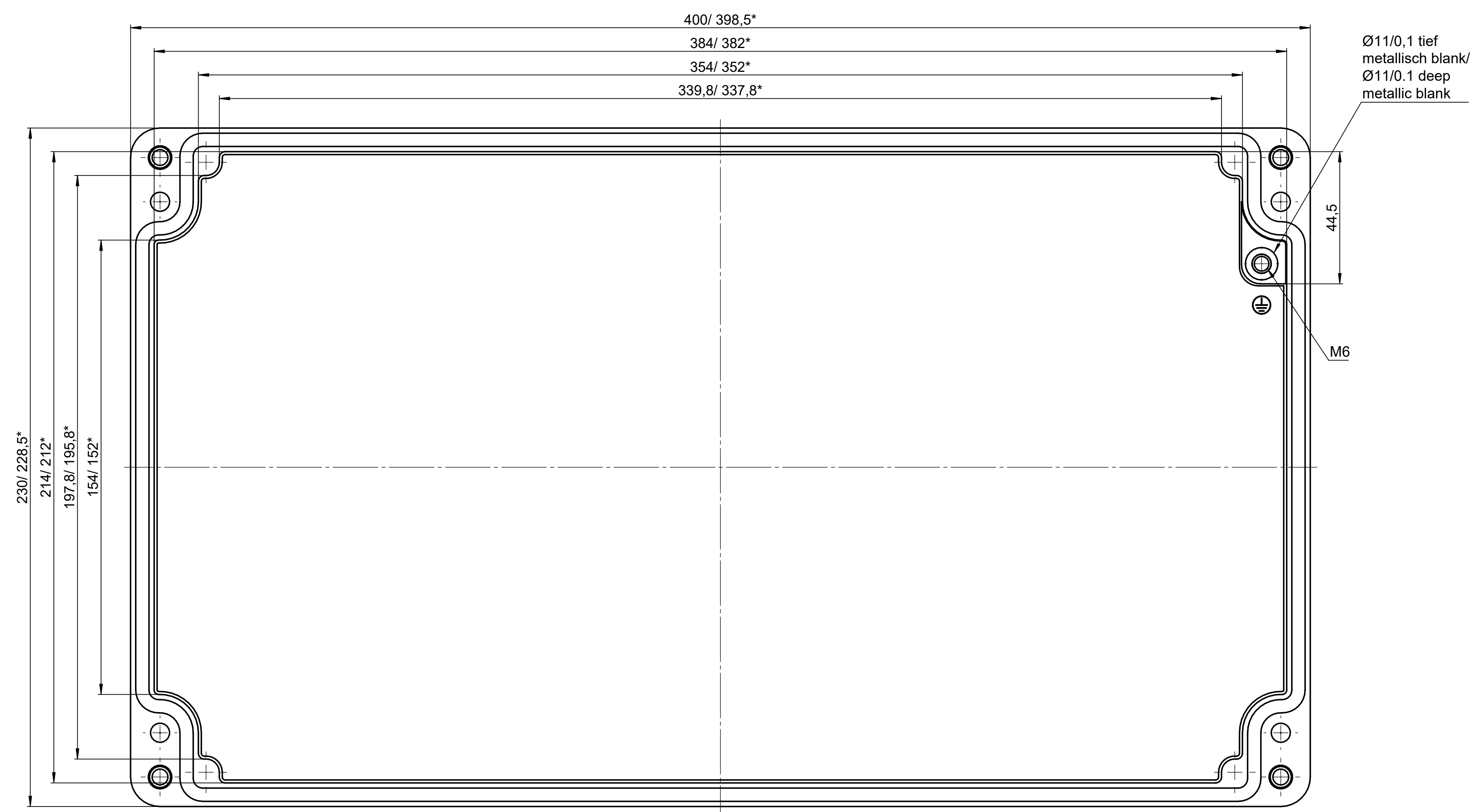
Deckel / Lid
