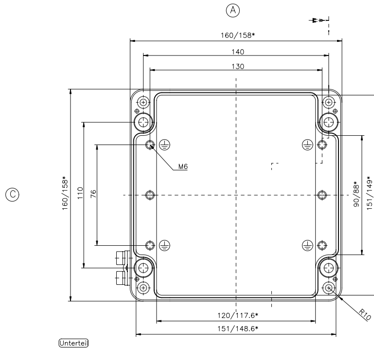
Unterteil
