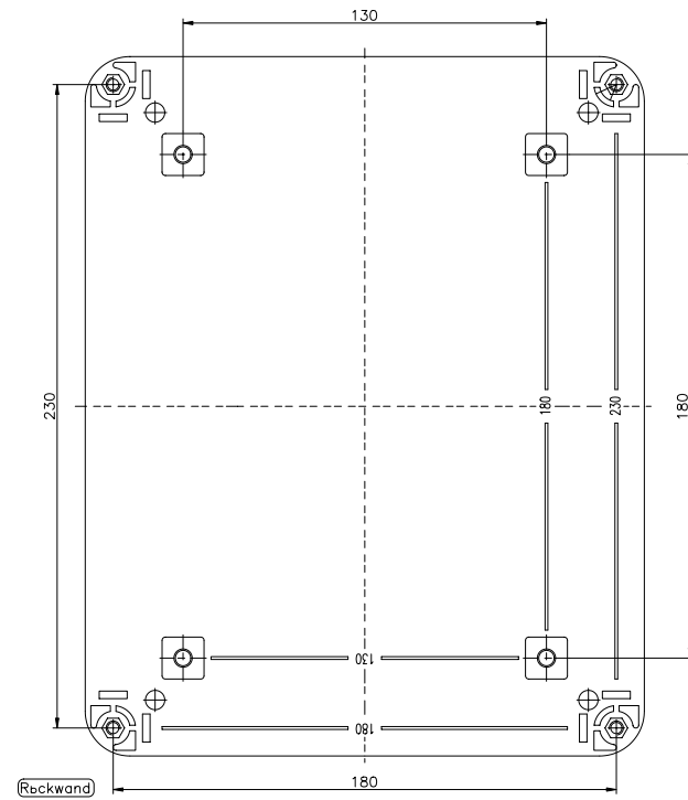
ABS- Gehguse mit Scharnierdeckel Best.Nr. 21.202590 / 22.202590
